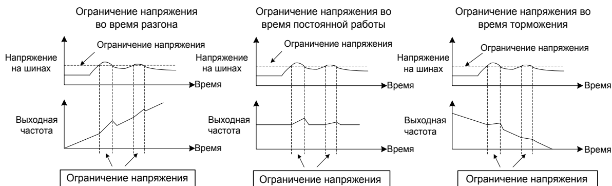
Рисунок 6-42 Ограничение напряжения
