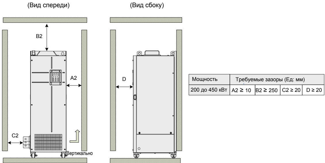
Рисунок 2-2 Правильные монтажные зазоры MD290T200G - MD290T450G и MD290T220P - MD290T500P
