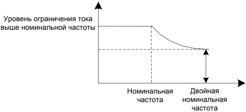
Рисунок 6-41 Ограничение тока выше номинальной частоты
