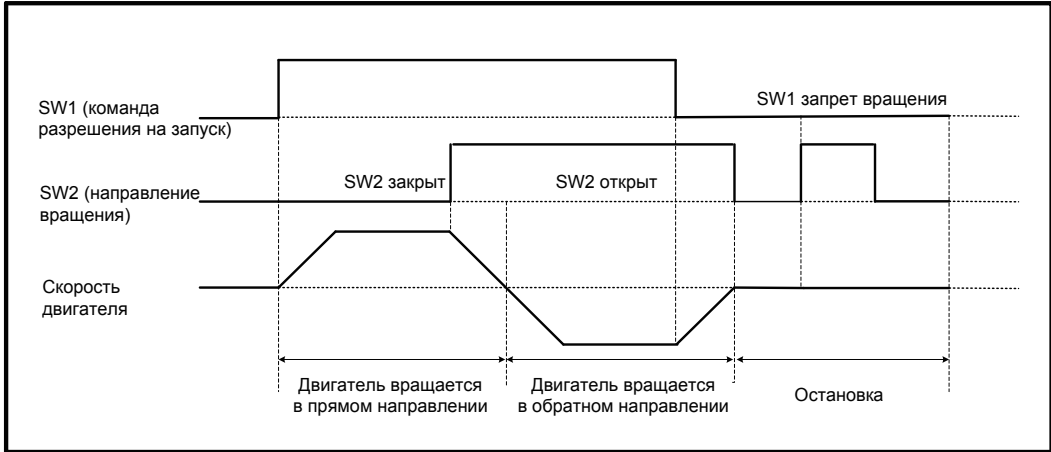
Рисунок 6-6 Последовательность двух-проводная 2
