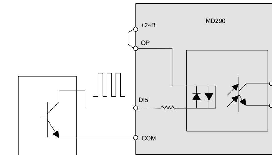
Рисунок 3-24 Подключение клеммы высокоскоростного импульсного входа
