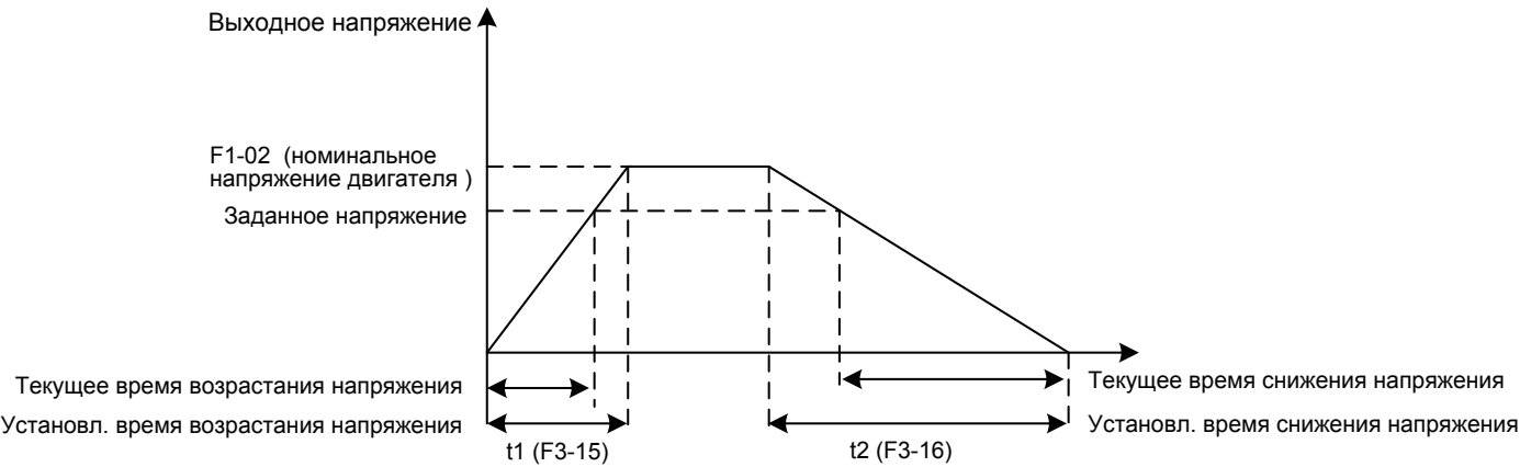
Рисунок 6-39 V/F разделение
