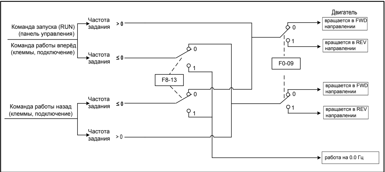
Рисунок 6-60 Управление запретом работы в обратном направлении
