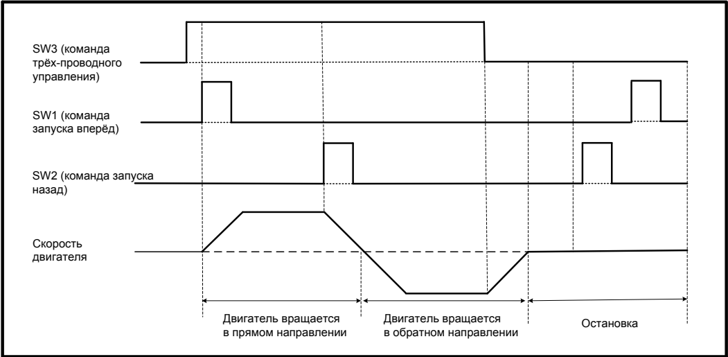
Рисунок 6-8 Последовательность трёх-проводная 1
