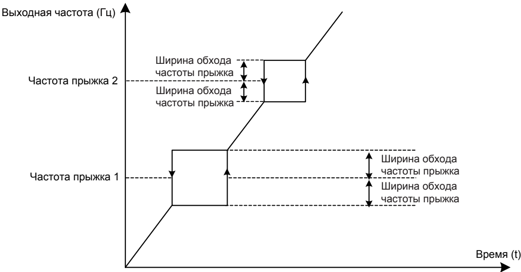
Рисунок 6-58 Частота прыжка
