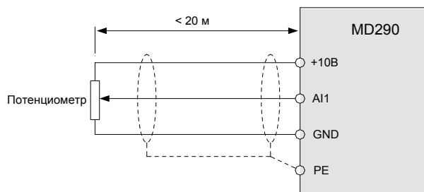
Рисунок 3-18 Подключение аналогового входа 1
