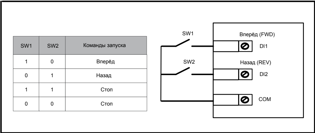
Рисунок 6-2 Схема подключения последовательности двух-проводной 1
