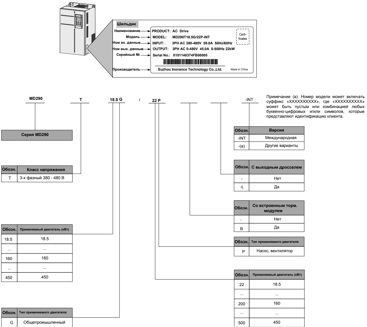
Рисунок 1-1 Идентификация типа изделия
