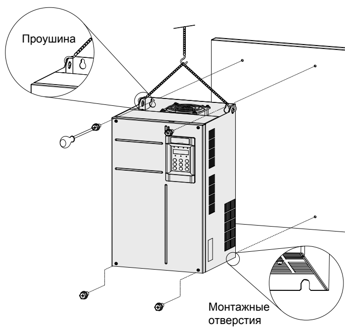
Рисунок 2-9 Настенный монтаж металлического корпуса
