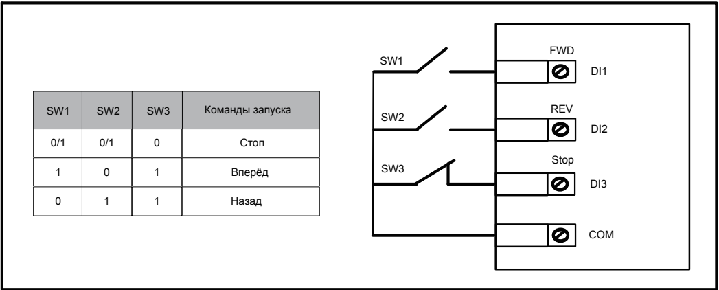
Диаграмма последовательности трёх-проводного режима управления 1
