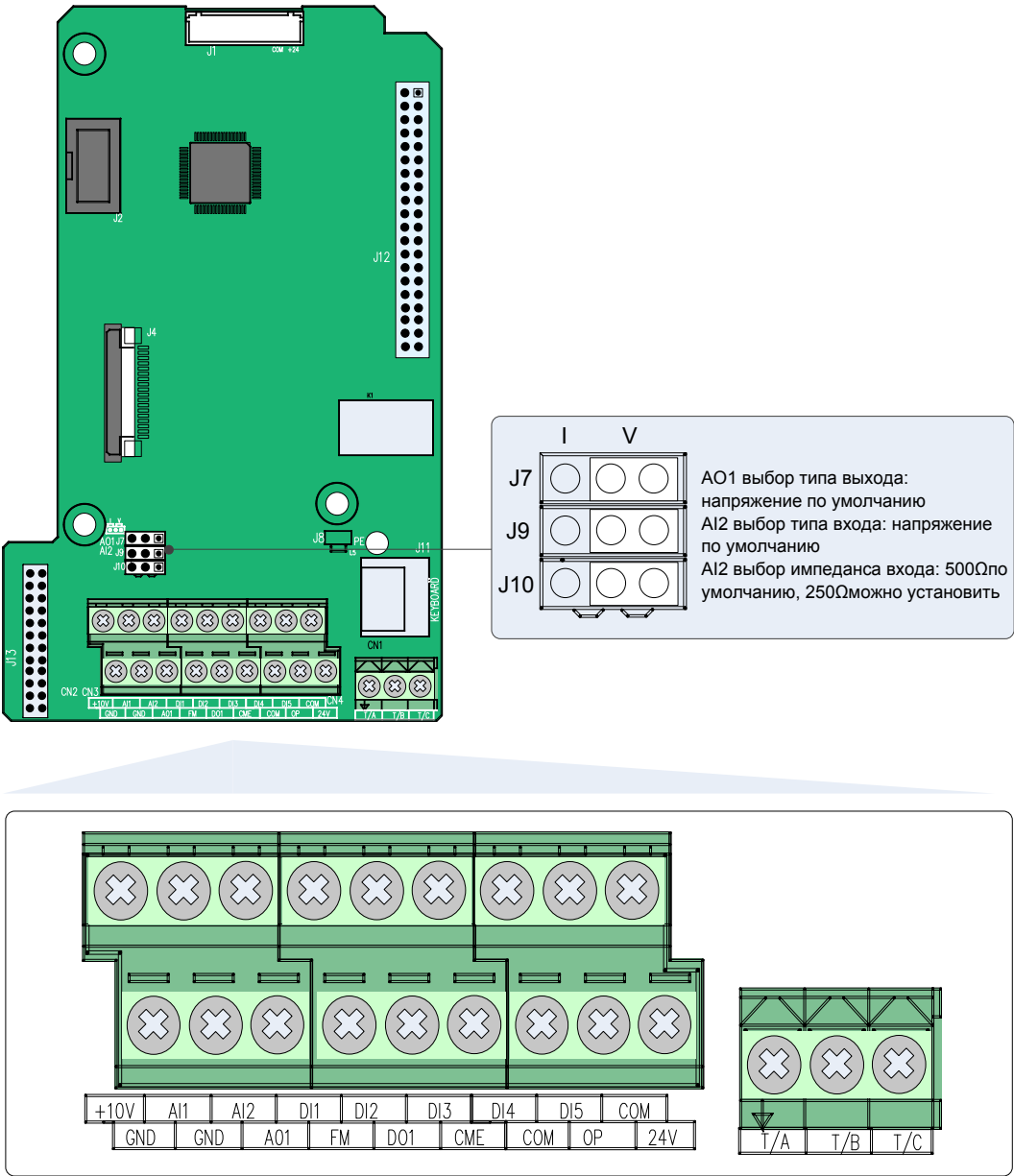
Рисунок 3-17 Расположение клемм цепи управления
