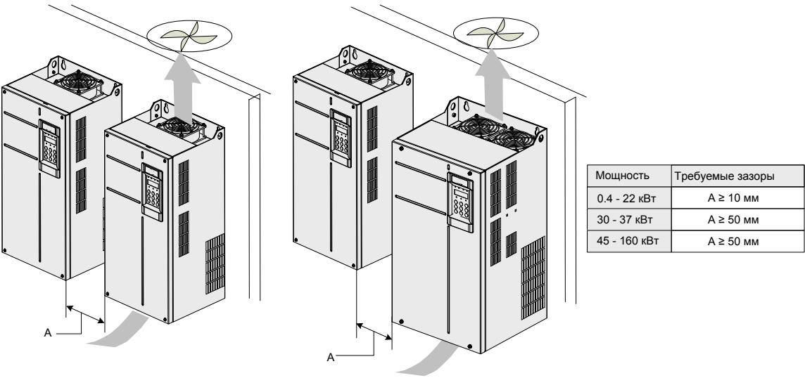
Рисунок 2-3 Зазор при установке нескольких приводов
