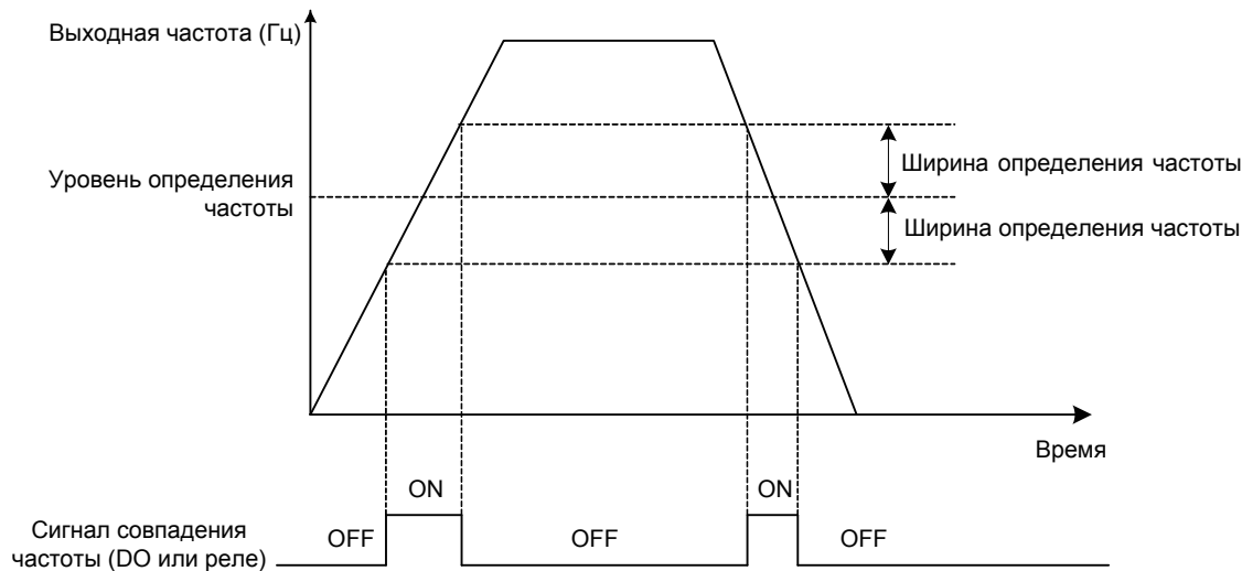
Рисунок 6-64 Определение совпадения частоты
