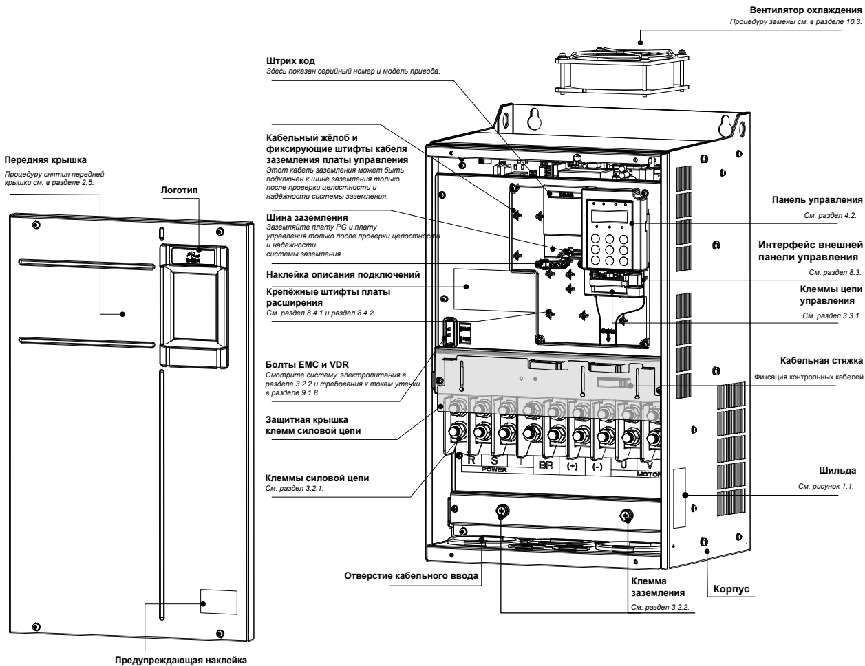
Рисунок 1-3 Внутренний вид MD290T45G/55PB ~ MD290T160G/200P (металлический корпус)
