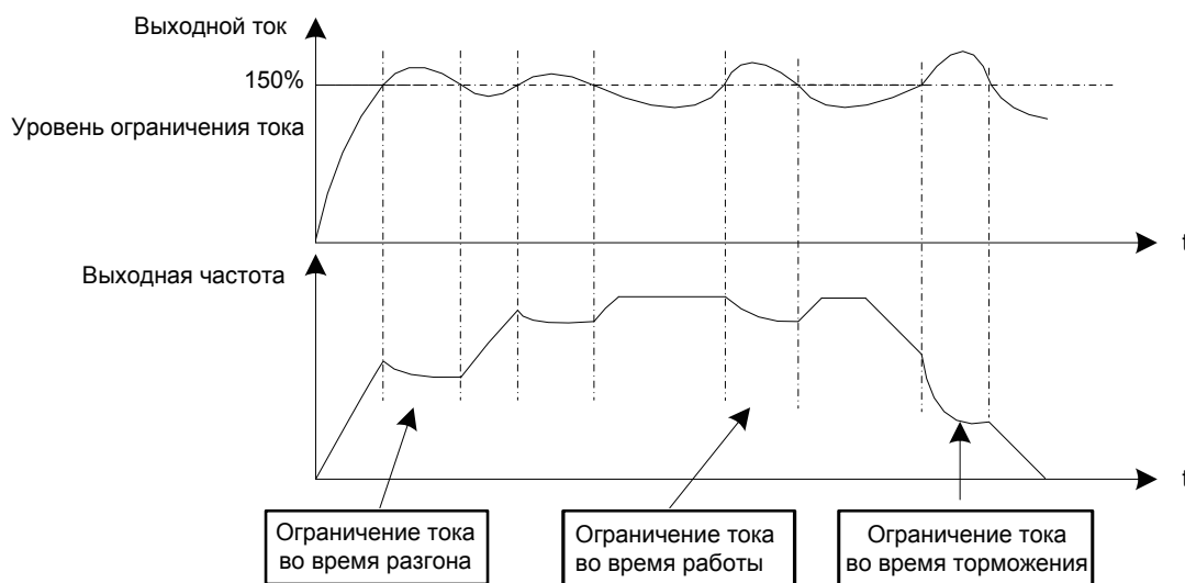
Рисунок 6-40 Ограничение тока
