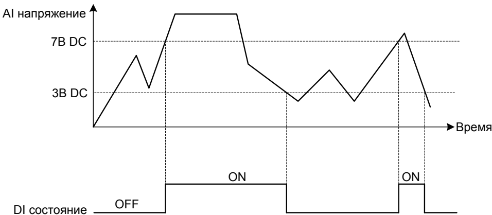
Рисунок 6-56 Взаимосвязь между входным напряжением AI и состоянием DI
