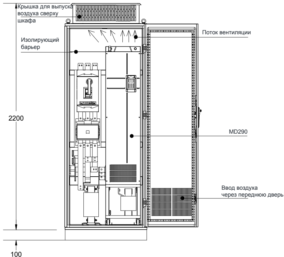
Рисунок 2-10 Шкаф без вентилятора сверху
