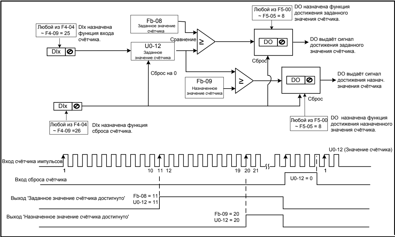
Рисунок 6-51 Функция счетчика
