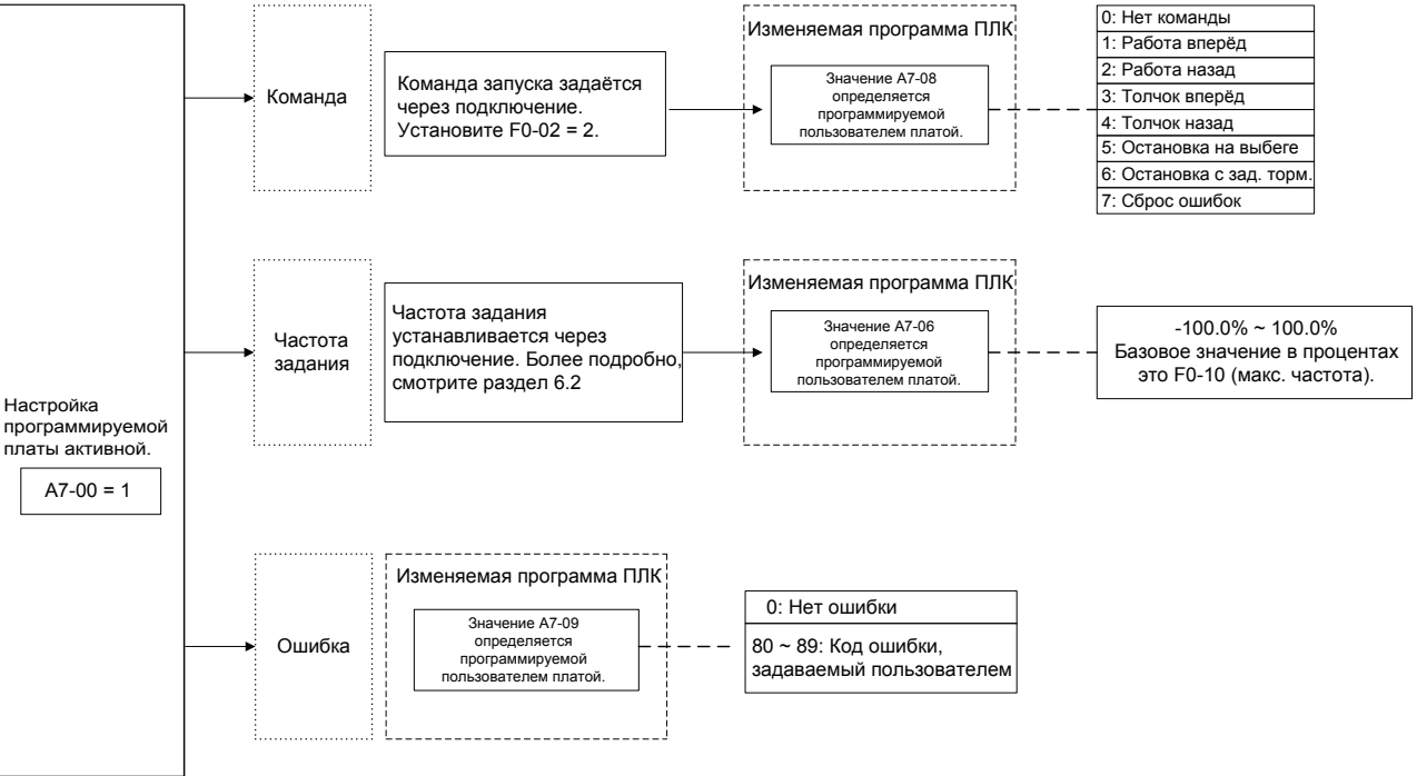
Рисунок 6-54 Программируемые пользователем функции (3)
