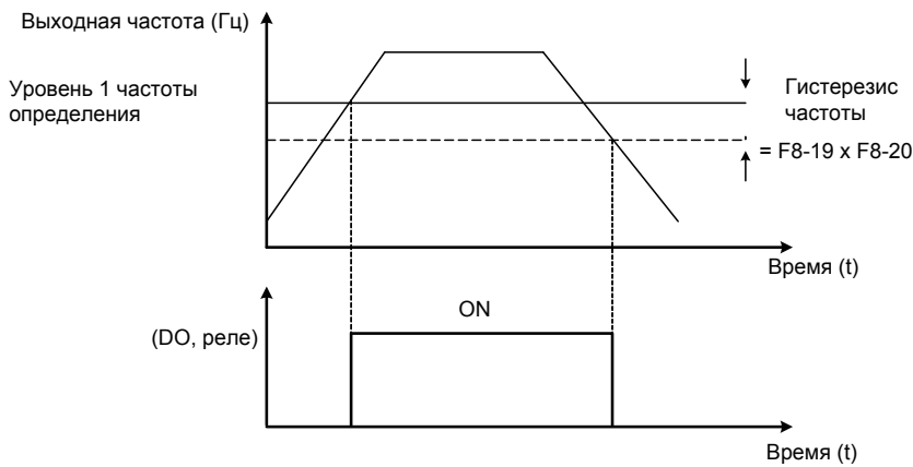
Рисунок 6-61 Определение частоты
