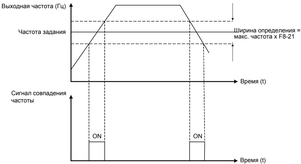
Рисунок 6-62 Ширина определения совпадения с частотой задания
