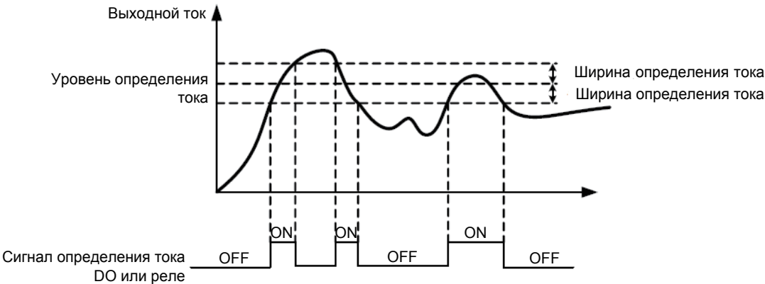
Рисунок 6-66 Определение тока
