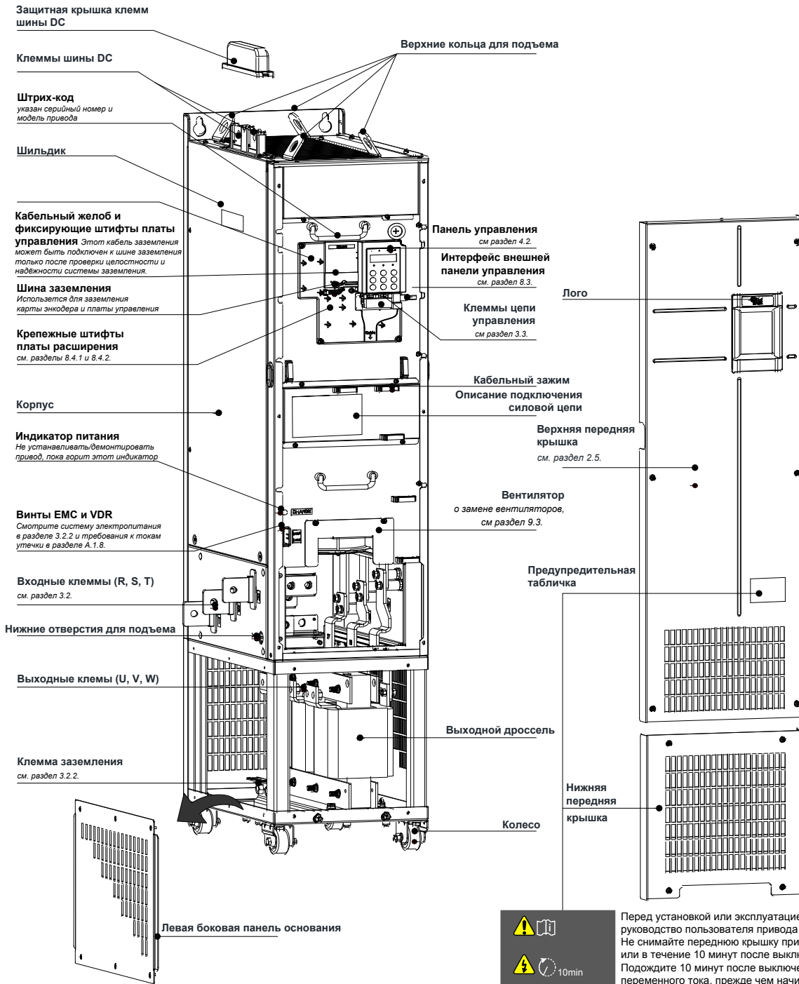
Рисунок 1-5 Внутренний вид MD290T200G-L - MD290T450G-L и MD290T220P-L - MD290T500P-L
