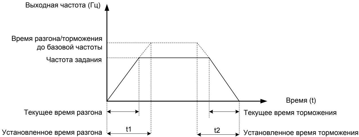
Рисунок 6-35 Время разгона/торможения
